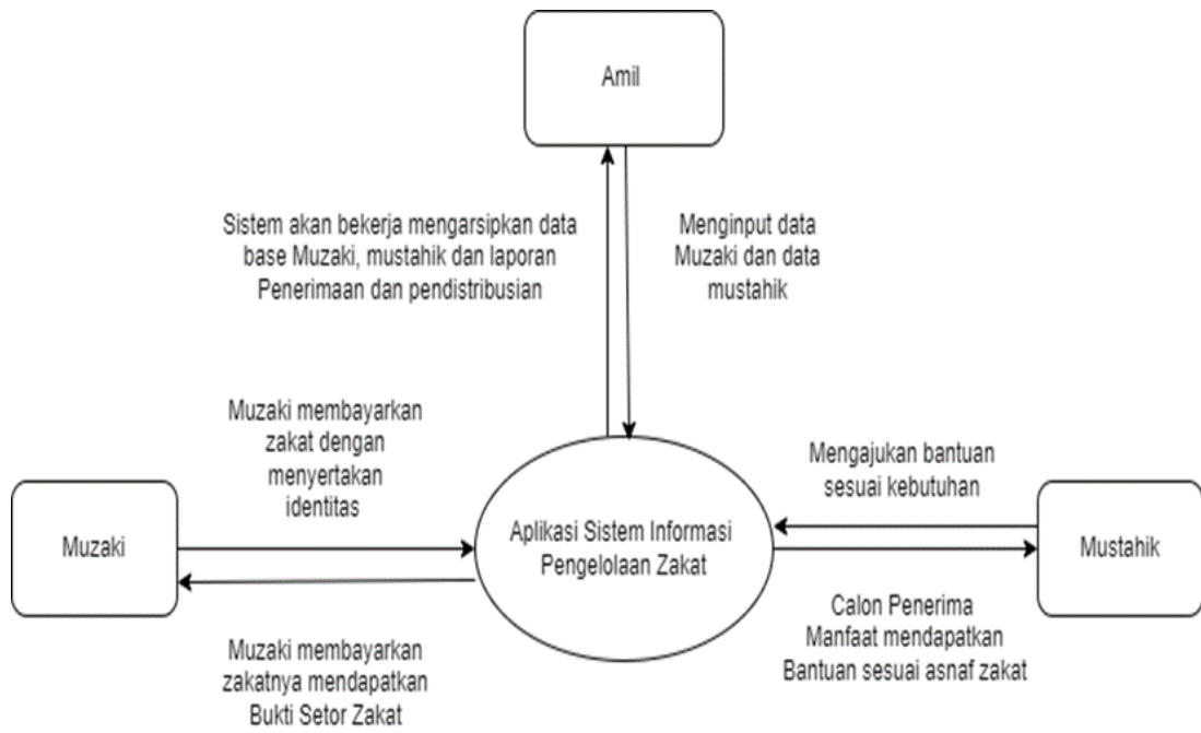
Gambar 4. Diagram Konteks
